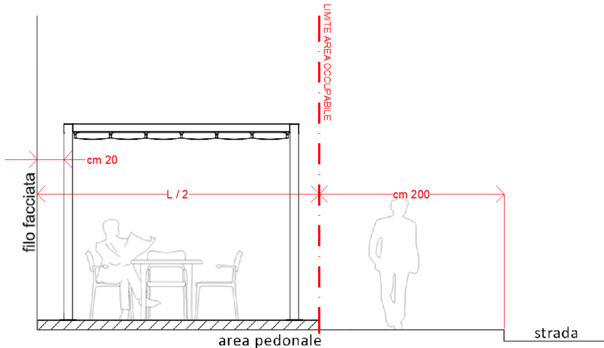
Schema dimensionale di riferimento - Vista frontale
