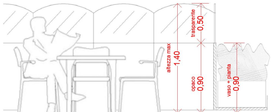
Schema dimensionale di riferimento - Sezione
