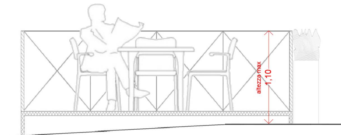
Schema dimensionale di riferimento - Sezione
