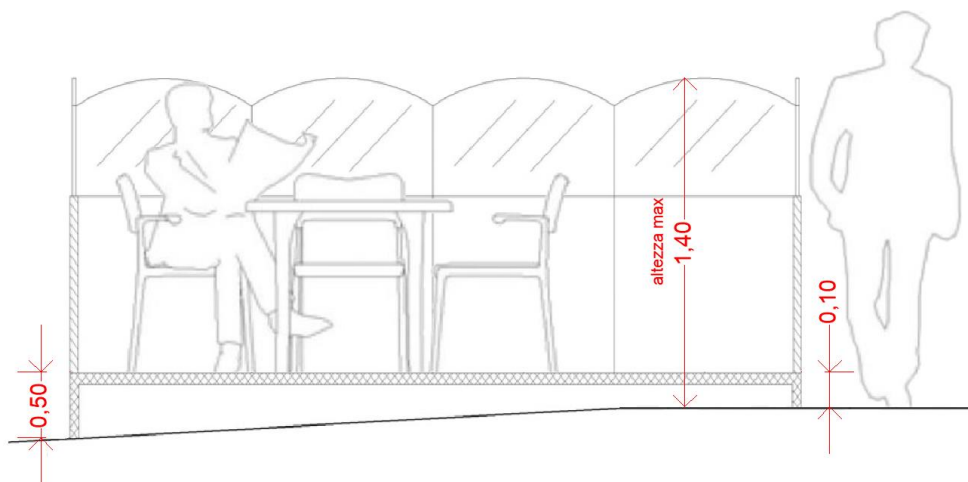
Schema dimensionale di riferimento - Sezione
