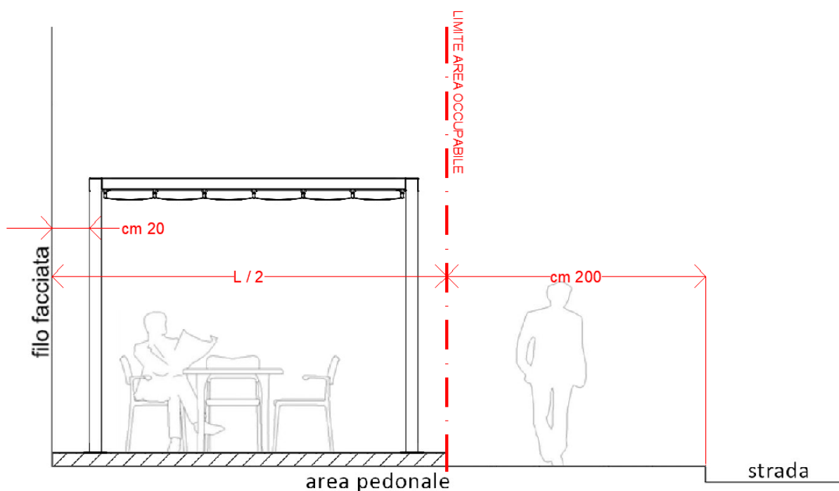
Schema dimensionale di riferimento - Vista frontale
