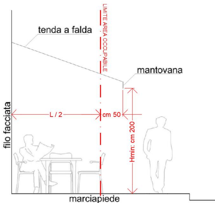
Schema dimensionale di riferimento - Vista frontale
