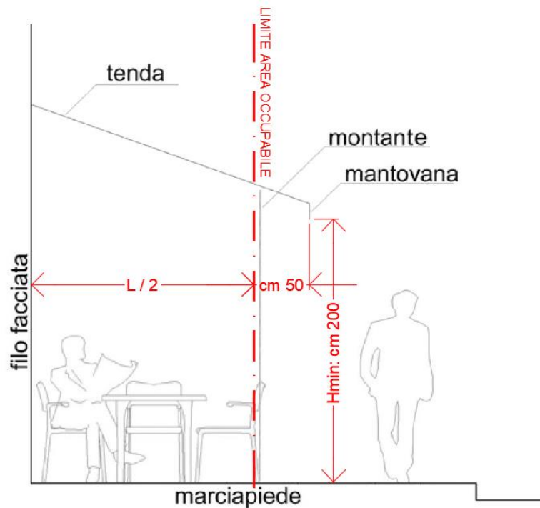
Schema dimensionale di riferimento - Vista frontale
